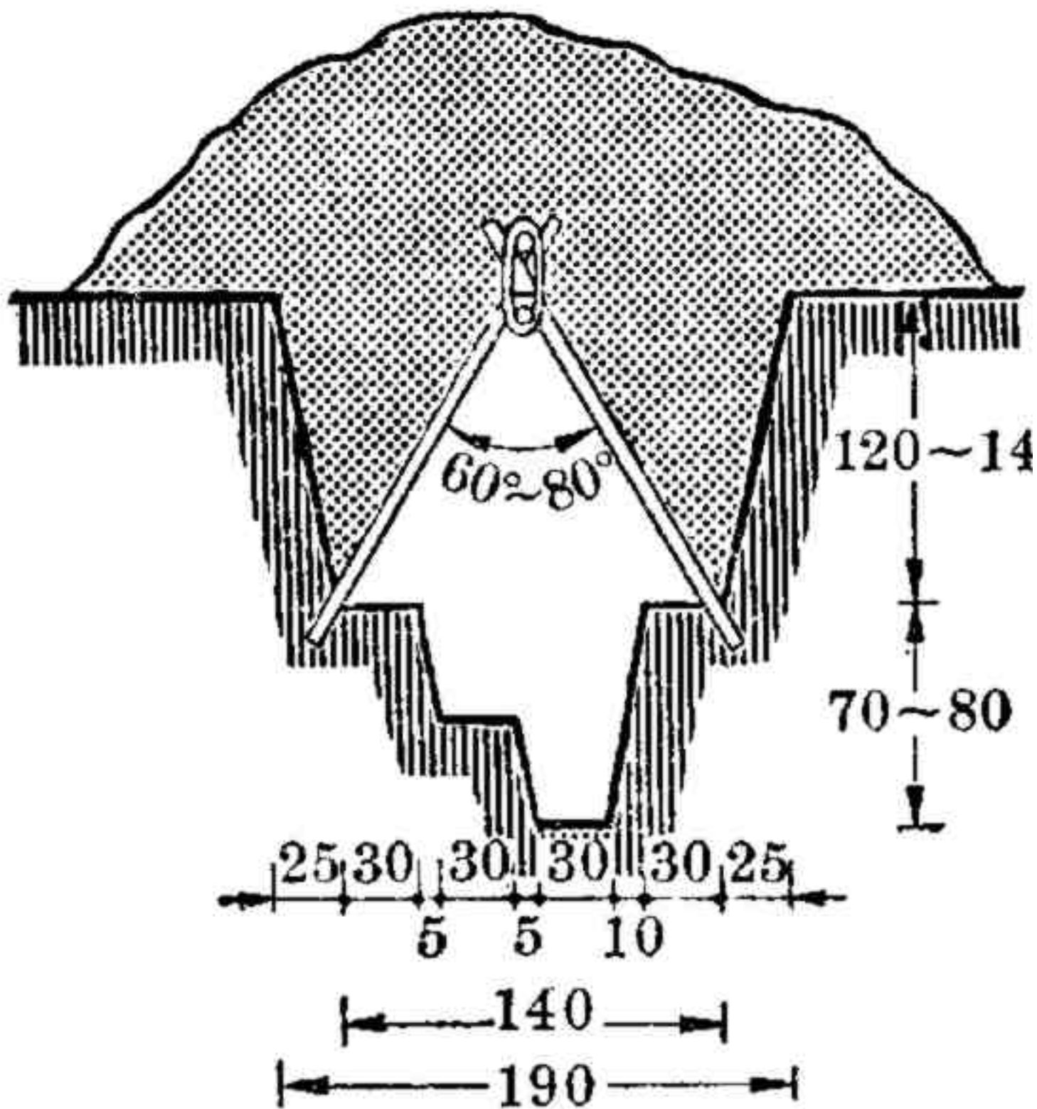
图 3-107 人字形骨架避弹所
